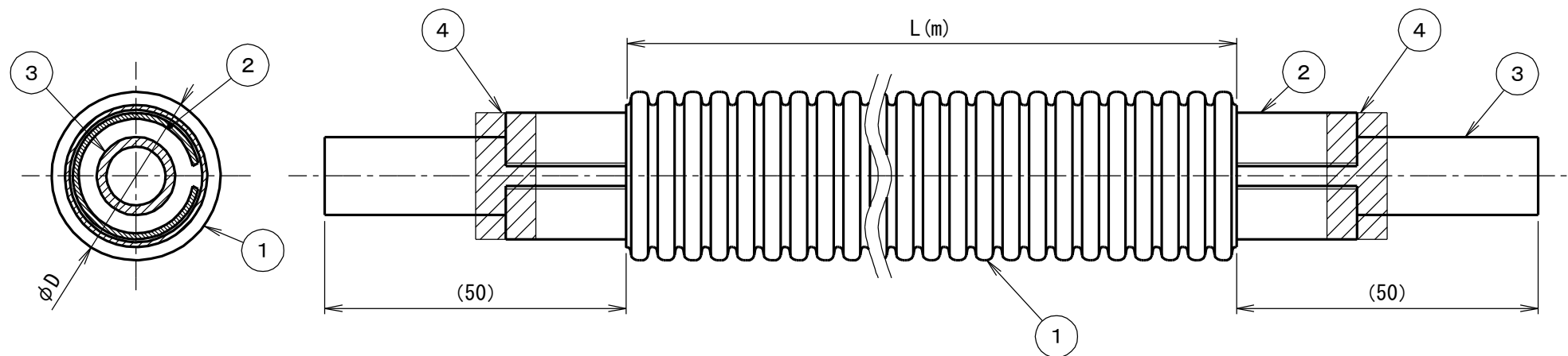
樹脂管寸法
